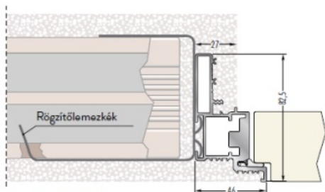
Tokszerkezet vakolt falhoz
