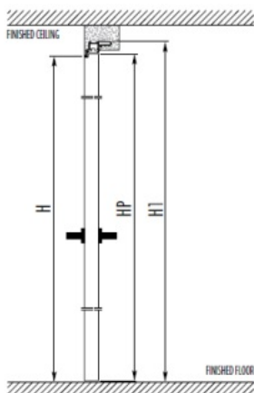
Tokszerkezet keresztartóval
