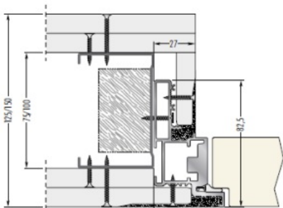
Tokszerkezet gipszkarton falhoz két lemezzel A kész fal vastagsága 125/150 mm
