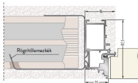
Tokszerkezet vakolt falhoz
