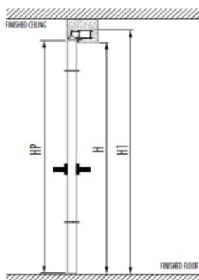
Tokszerkezet keresztartóval
